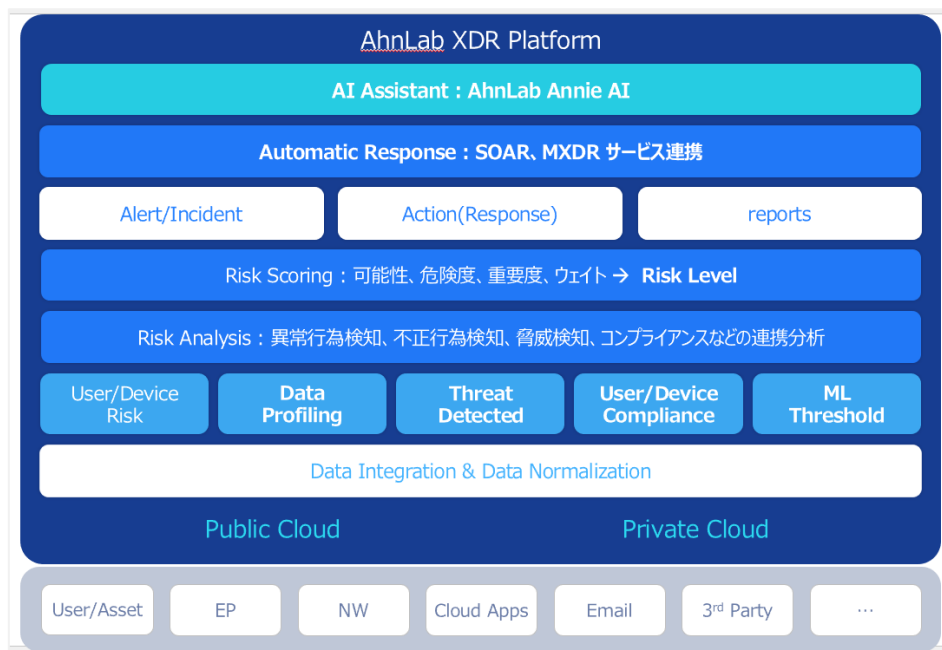
【図1】「AhnLab XDR」プラットフォーム構造図
